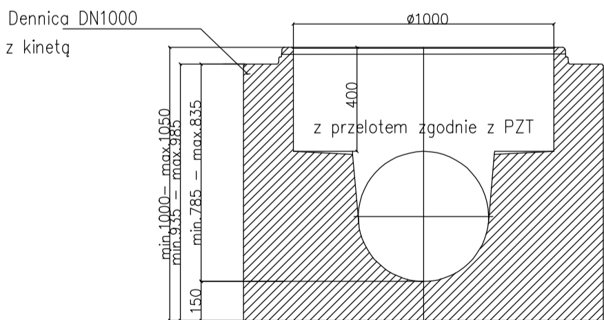
PRZEKRÓJ E-E
