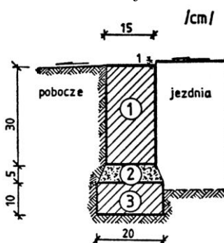
f) Krawężnik typu drogowego 15 × 30 cm na ławie betonowej
