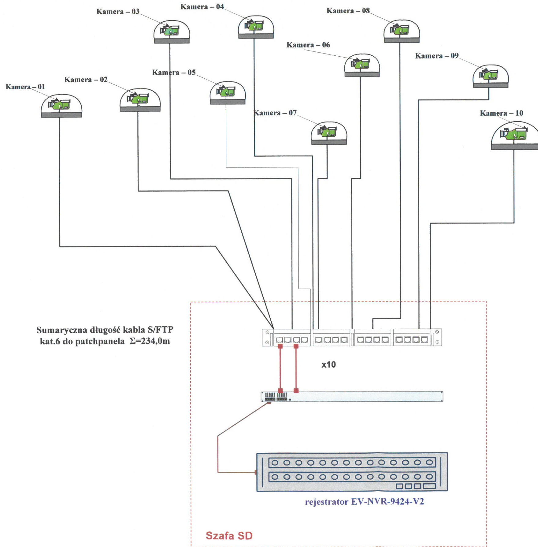
Schemat ideowy połączeń sieci monitorowania CCTV warsztatów szkolnych w Zespole Szkół Zawodowych w Szprotawie
