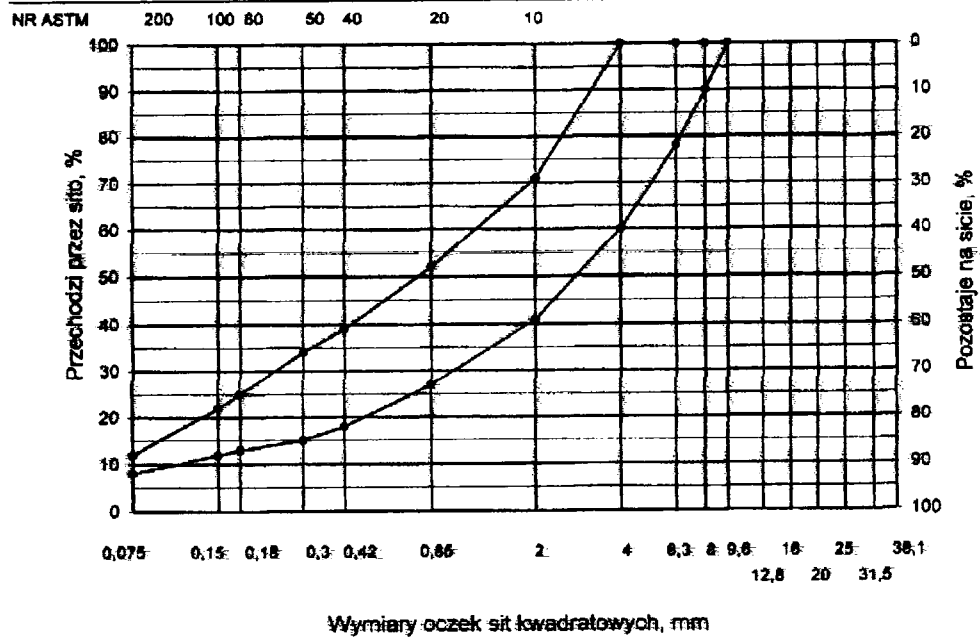
Rys. 3. Krzywe graniczne uziarnienia mieszanki mineralnej BA od 0 do 8mm, od 0 do 6,3 mm do warstwy ścierniej nawierzchni drogi o obciążeniu ruchem nawierzchni drogi o obciążeniu ruchem KR1 lub KR2
