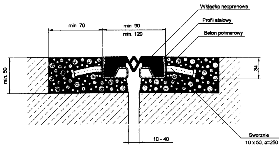
Rys. 1. Urządzenie dylatacyjne ze sworzniami
