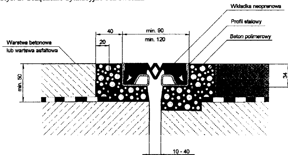
Rys. 2. Urządzenie dylatacyjne bez sworzni
