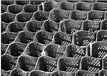
Rys. 7. Ułożona i wypełniona geosiatka komórkowa a) Geosiatka po ułożeniu, b) Geosiatka przymocowana do podłoża kotwami i częściowo zasypana, c) Geosiatka całkowicie zasypana kruszywem
