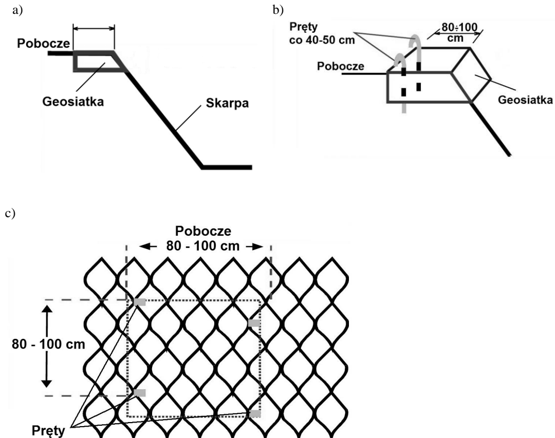
Rys. 12. Umocnienie skarpy geosiatką komórkową
