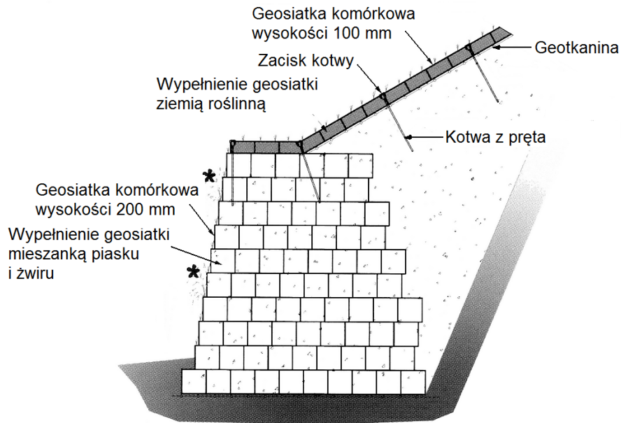
Rys. 11. Zakotwienie górnej części geosiatki komórkowej na poboczu drogi przy umocnieniu skarpy nasypu a) Schemat skarpy nasypu z miejscem zakotwienia geosiatki na poboczu drogi b) Górna część geosiatki komórkowej jest ułożona na szerokości 80÷100 cm pobocza drogi z przymocowaniem prętami stalowymi w kształcie litery J c) Widok z góry geosiatki na poboczu i części skarpy
