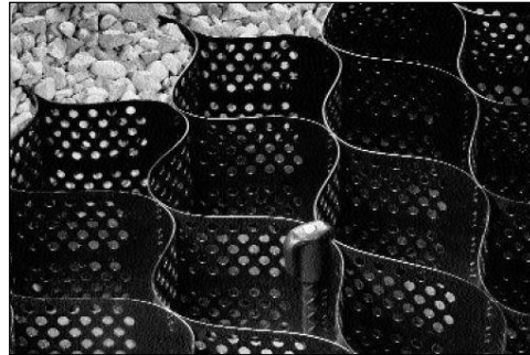
Rys. 7. Ułożona i wypełniona geosiatka komórkowa a) Geosiatka po ułożeniu, b) Geosiatka przymocowana do podłoża kotwami i częściowo zasypana, c) Geosiatka całkowicie zasypana kruszywem
