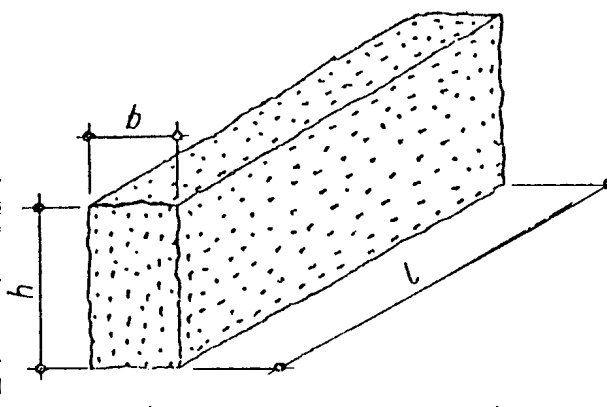
Tablica 4. Wymiary krawężników drogowych
