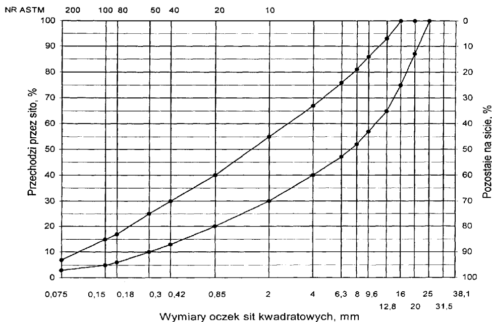
Rys. 8. Krzywe graniczne uziarnienia mieszanek mineralnej BA od 0 do 20 mm do warstwy wiążącej, wyrównawczej i wzmacniającej nawierzchni drogi o obciążeniu ruchem KR1 lub KR2
