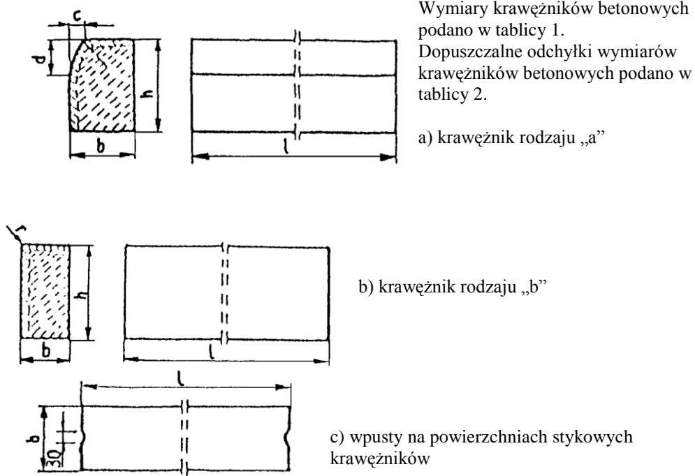
Rys. 1. Wymiarowanie krawężników
