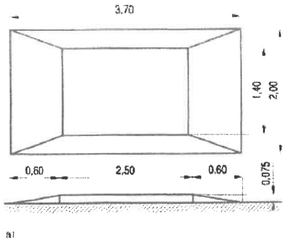
Rys. 8 1.6. Przykłady progów zwalniających wyspowych
