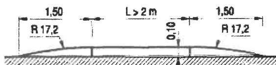
Rys. 8.1.2. Liniowy próg zwalniający płytowy U-16b o ograniczonej prędkości przejazdu 25–30 km/h
