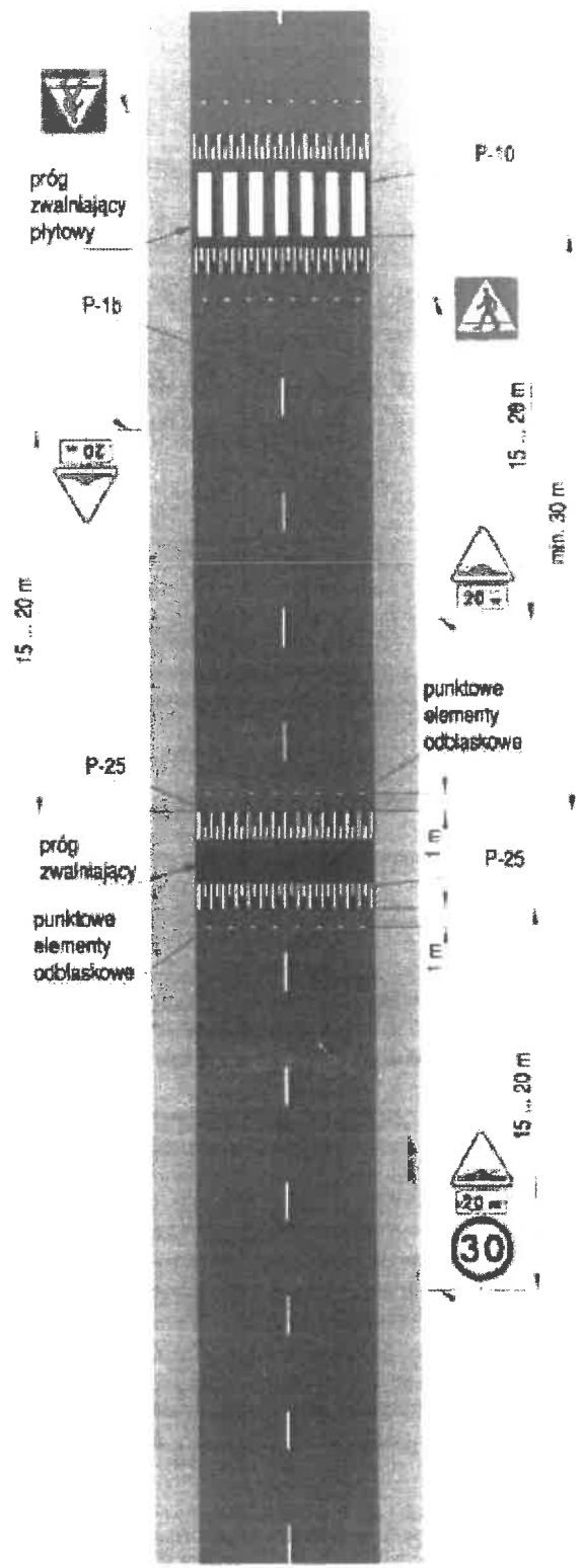
Rys. 8.1.7. Oznakowanie progów zwalniających U-16
