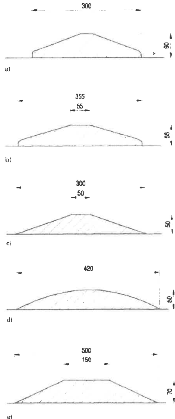
Rys. 8.2.1. Kształt i wymiary w przekroju poprzecznym przykładowych progów podrzutowych
