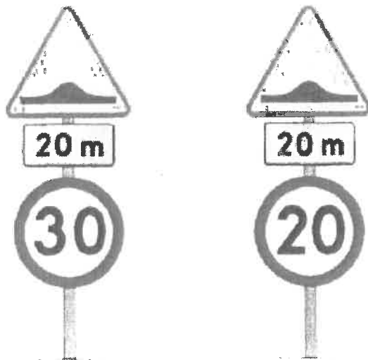
Rys. 8.1.8 Oznakowanie pionowe progów zwalniających:
