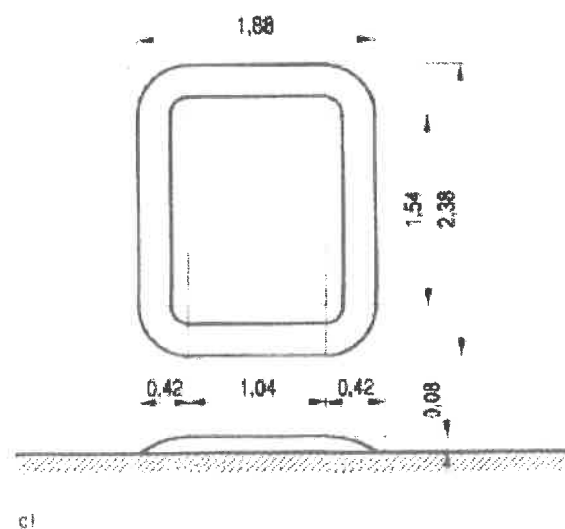
Rys. 8.1.7. Oznakowanie progów zwalniających U-16
