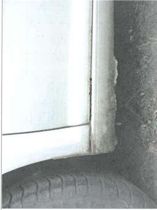
Foto 32 – skorodowane poszycie drzwi oraz skorodowany próg drzwiowy
